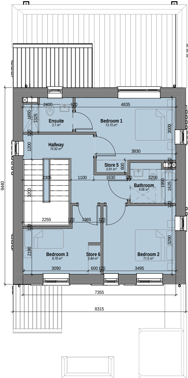
3 DAD - Level 02 Scale: 1 : 100
