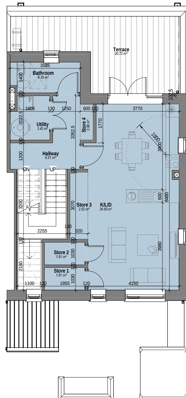
2 DBE - Level 01 Scale: 1 : 100
