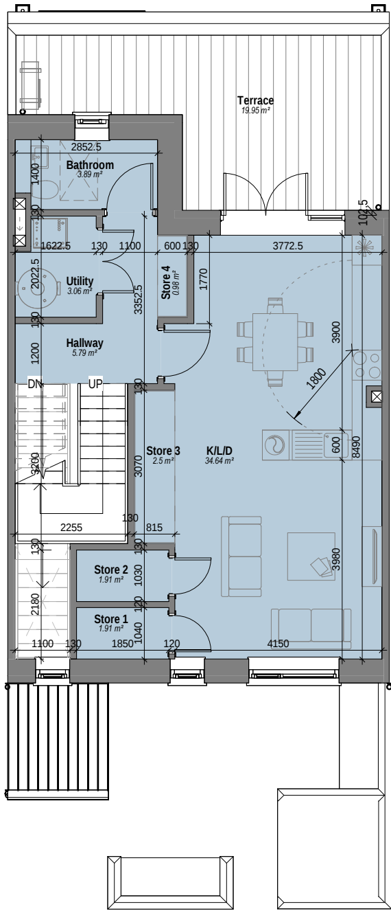
2 DAM - Level 01 Scale: 1 : 100
