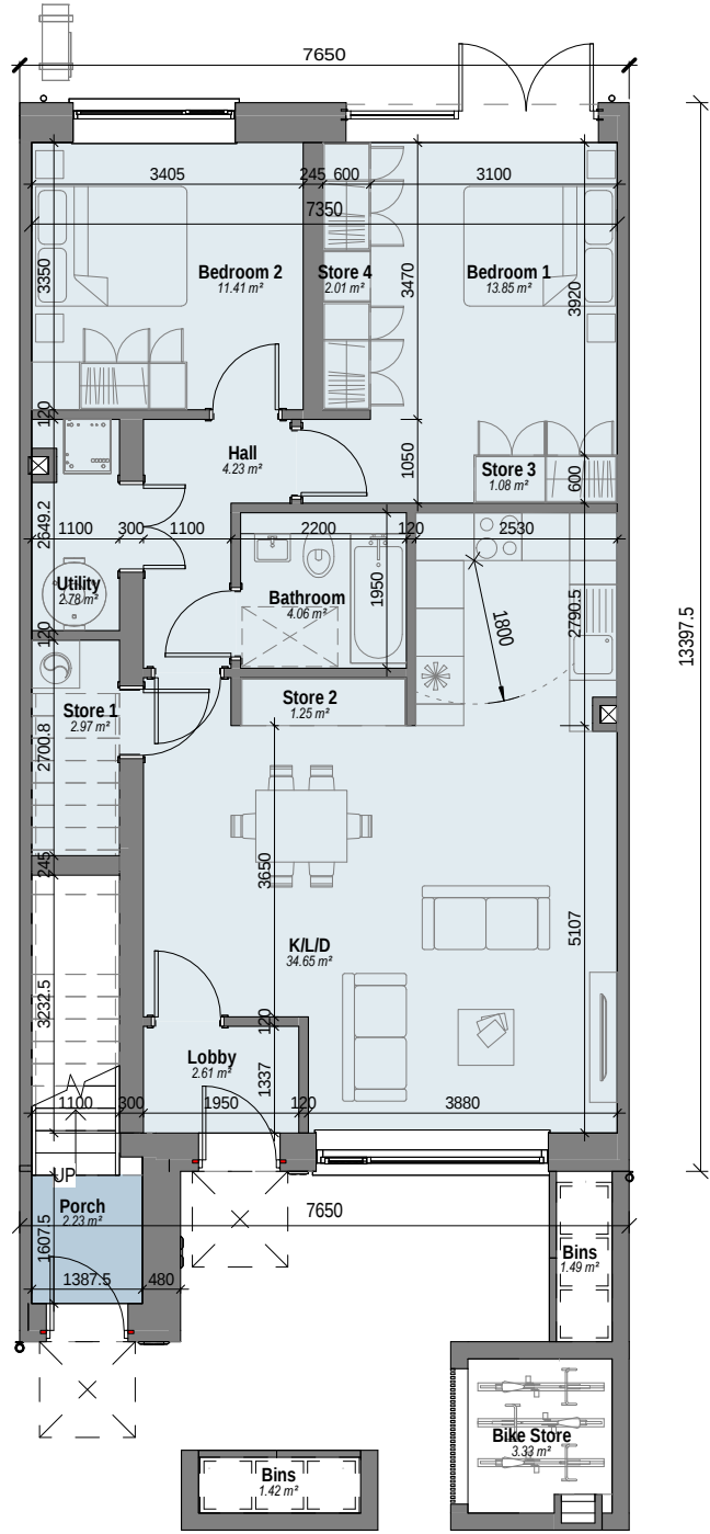
1 DCM - Level 00 Scale: 1 : 100
