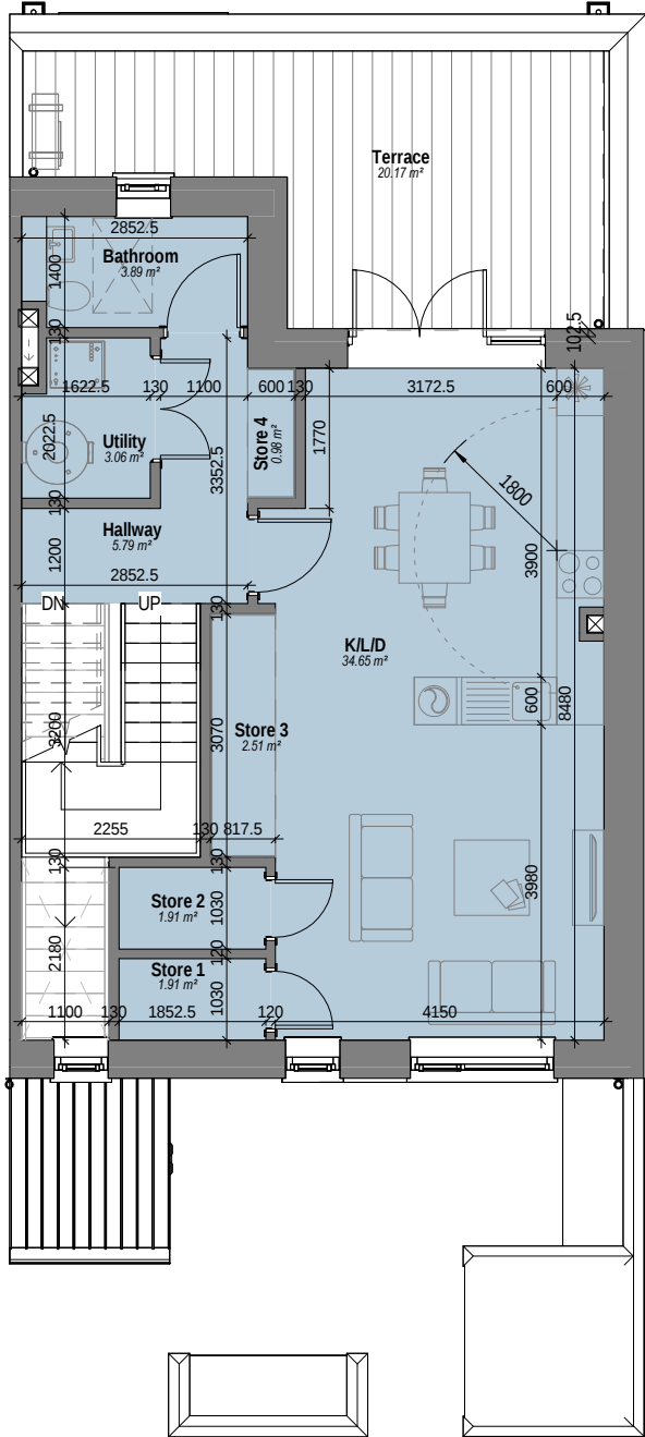
2 DCES - Level 01 Scale: 1 : 100
