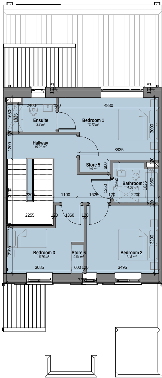
3 DAM - Level 02 Scale: 1 : 100
