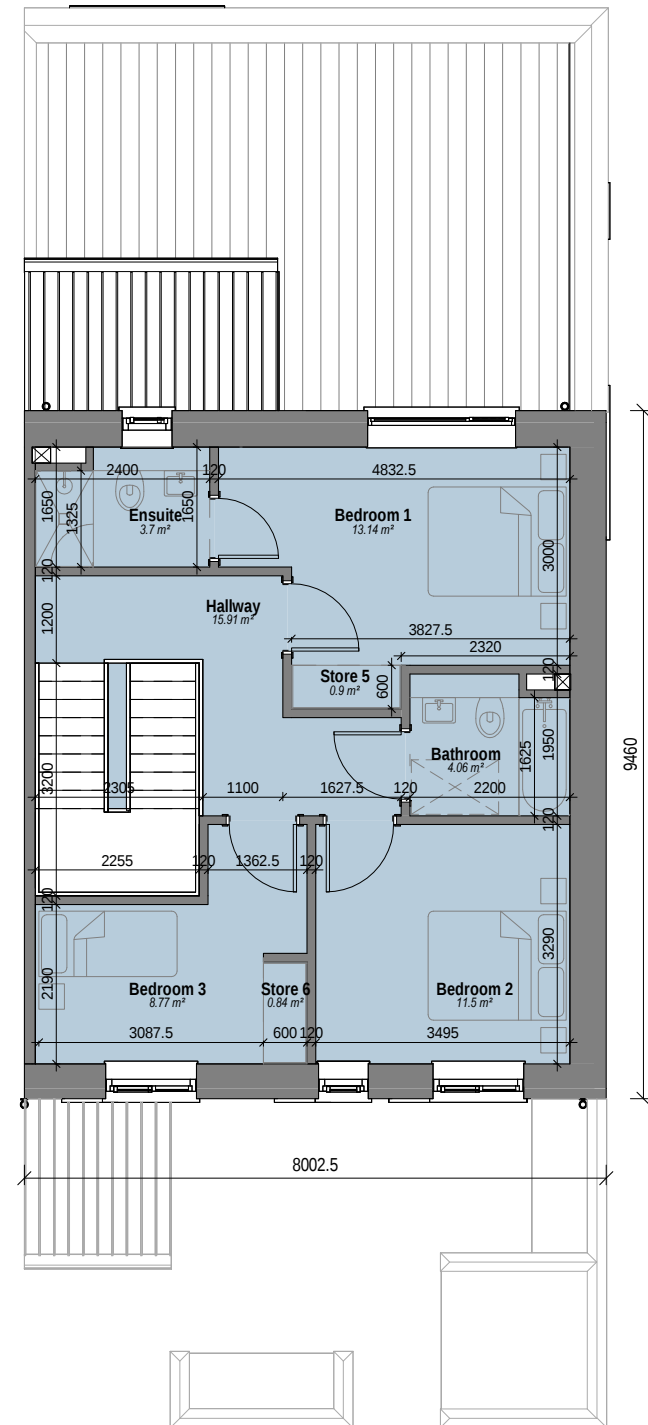
3 DDE - Level 02 Scale: 1 : 100
