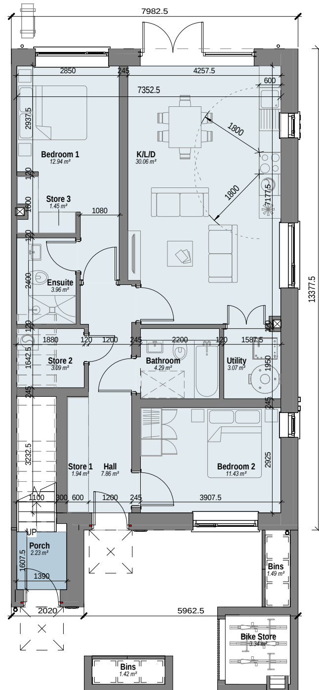
1 DAE - Level 00 Scale: 1 : 100
