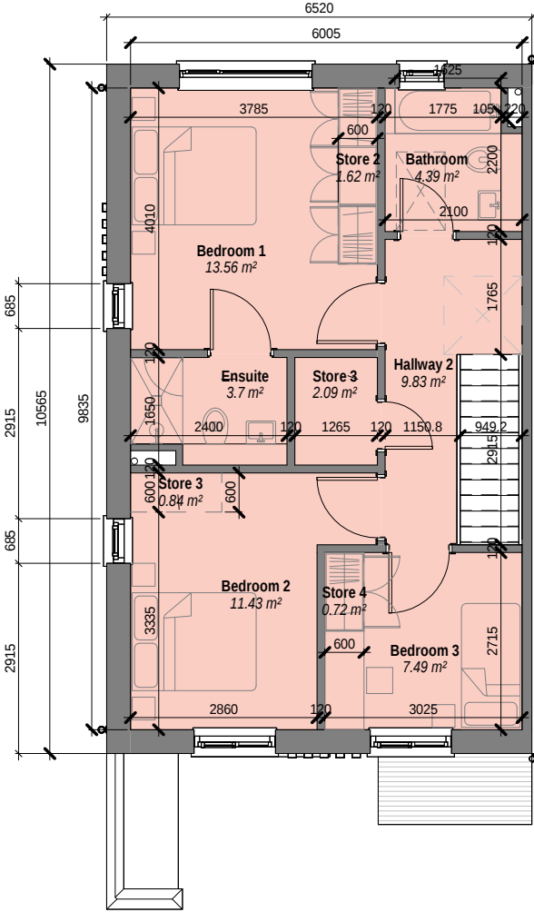
2 H3AE - Level 01 Scale: 1 : 100
