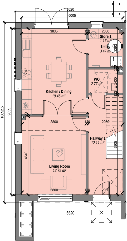
1 H3BE - Level 00 Scale: 1 : 100
