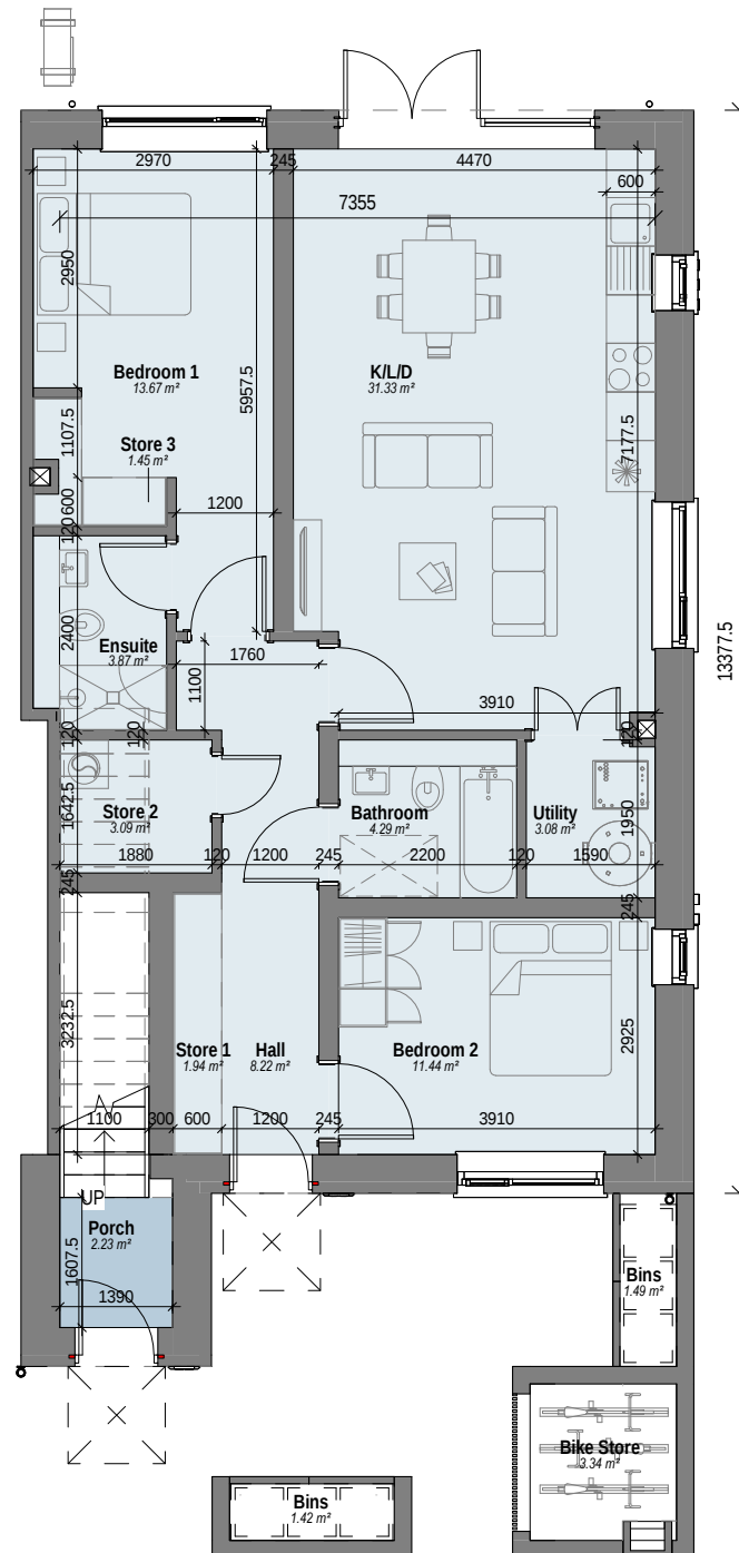
1 DBE - Level 00 Scale: 1 : 100
