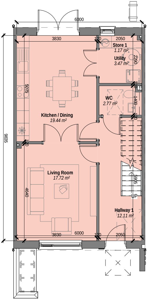
1 H3AM - Level 00 Scale: 1 : 100
