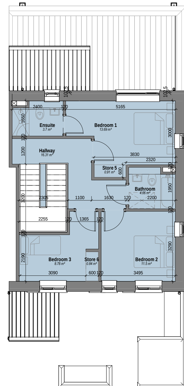
3 DBE - Level 02 Scale: 1 : 100
