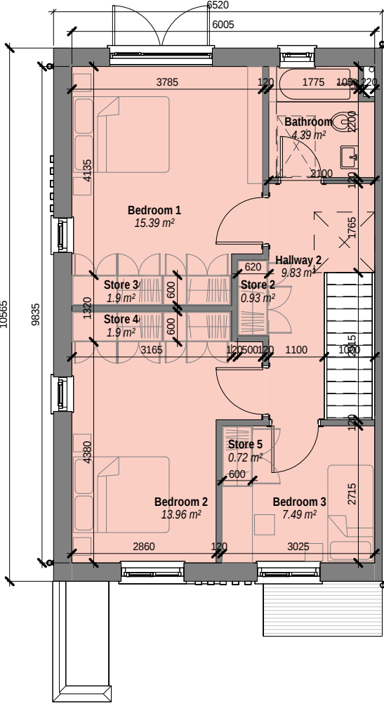
2 H3BE - Level 01 Scale: 1 : 100
