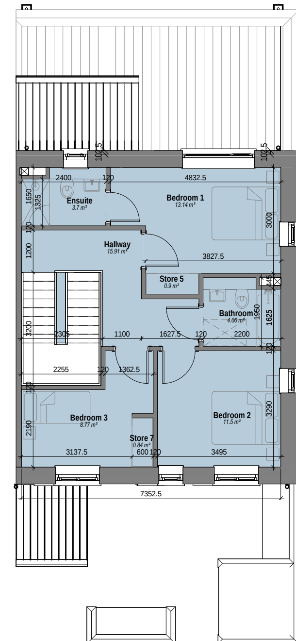
3 DAE - Level 02 Scale: 1 : 100
