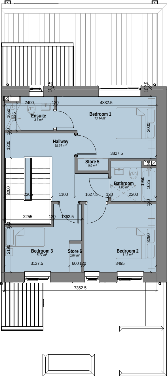
3 DCES - Level 02 Scale: 1 : 100
