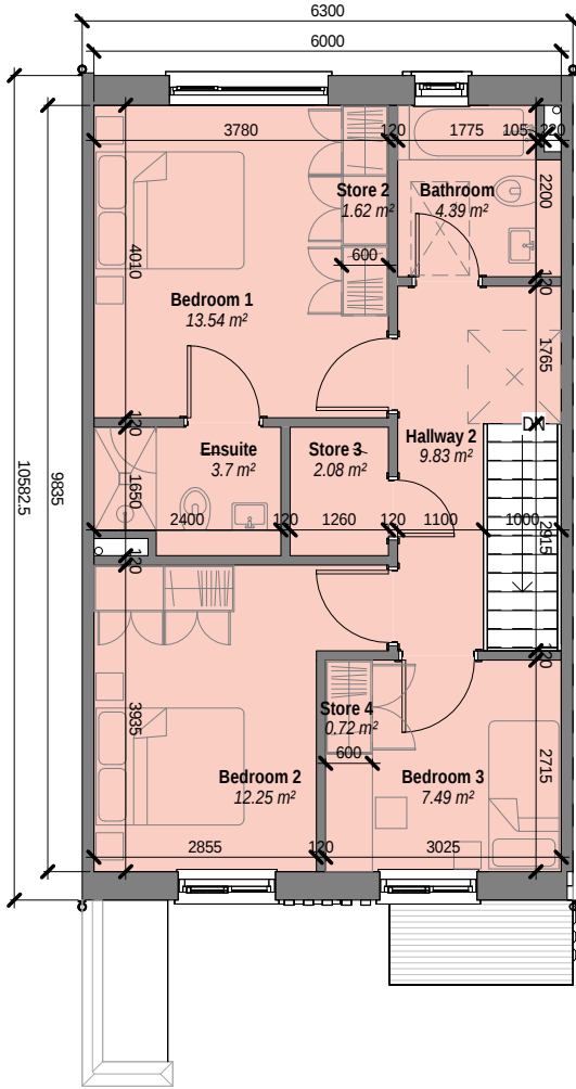
2 H3AM - Level 01 Scale: 1 : 100
