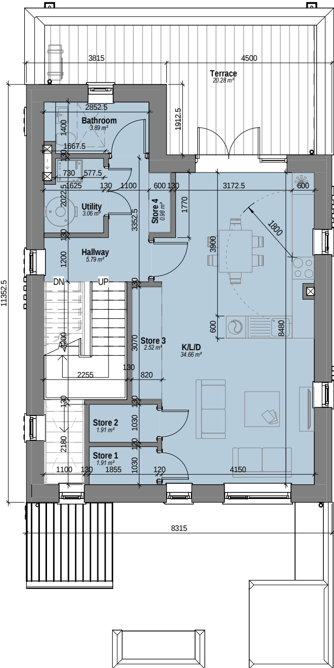
2 DAD - Level 01 Scale: 1 : 100
