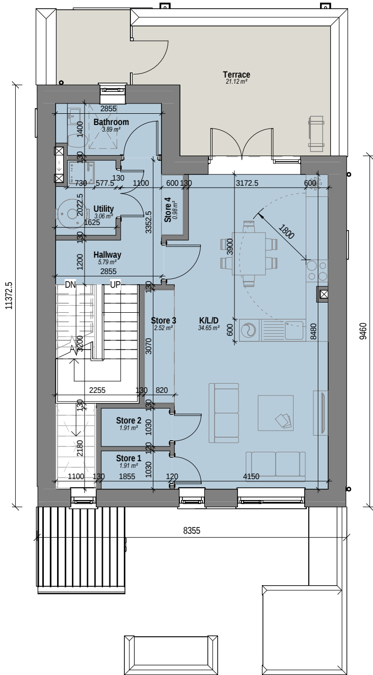
2 DCD - Level 01 Scale: 1 : 100
