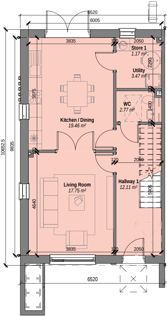
1 H3AE - Level 00 Scale: 1 : 100
