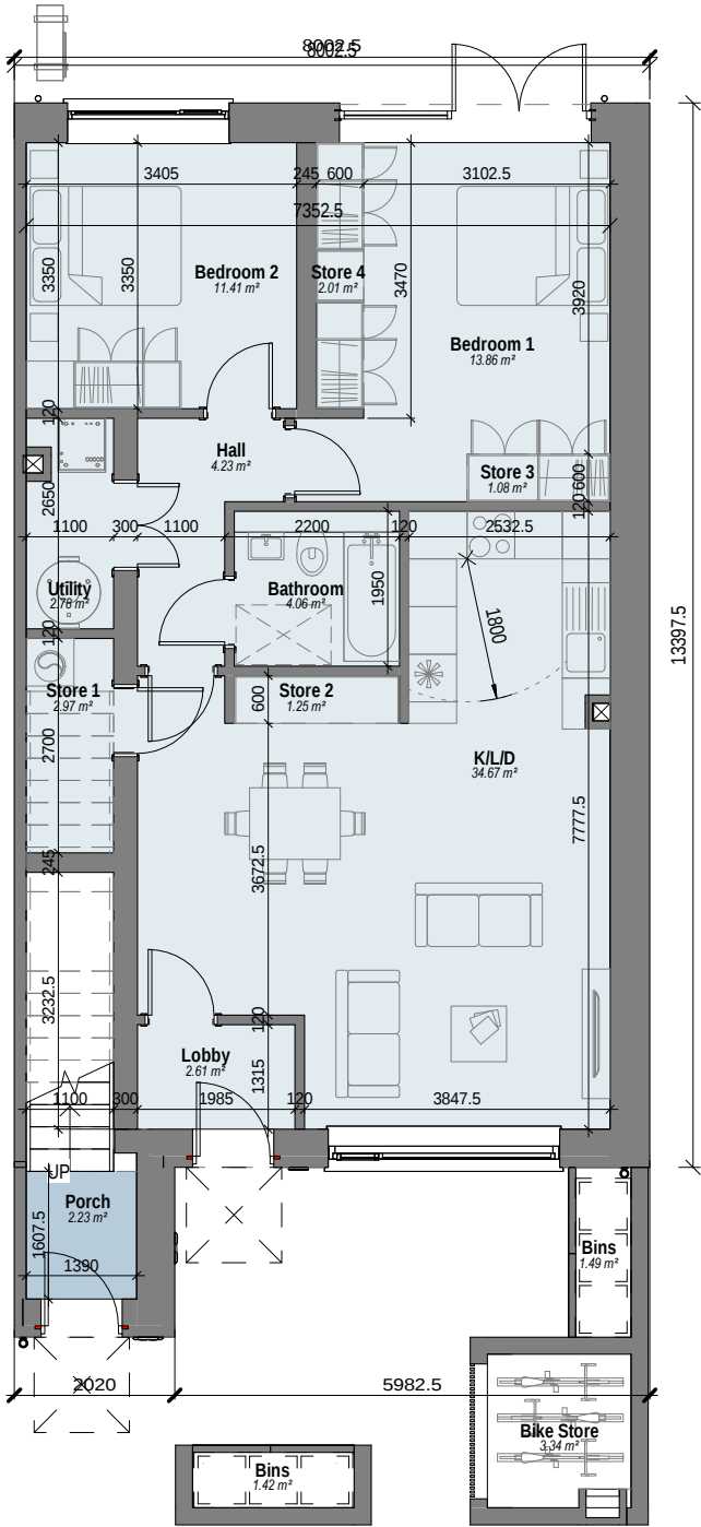
1 DCES - Level 00 Scale: 1 : 100
