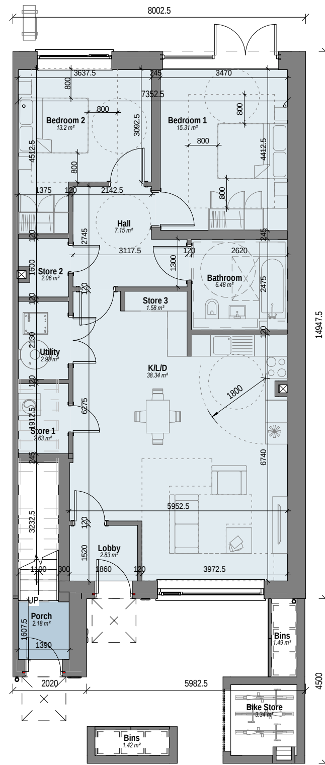
1 DEE - Level 00 Scale: 1 : 100
