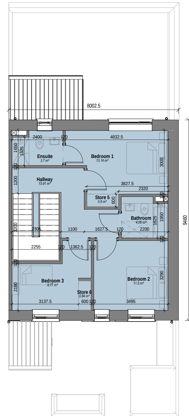
3 DEE - Level 02 Scale: 1 : 100
