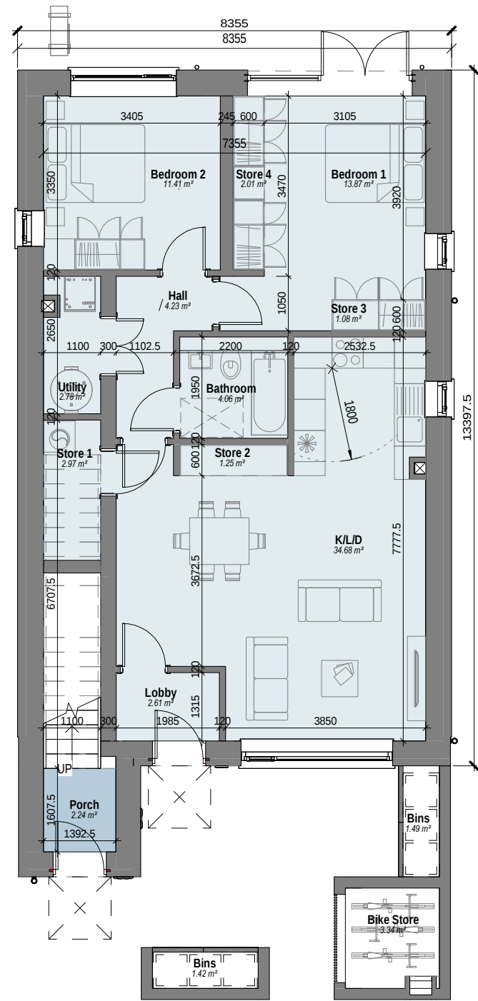
1 DCD - Level 00 Scale: 1 : 100
