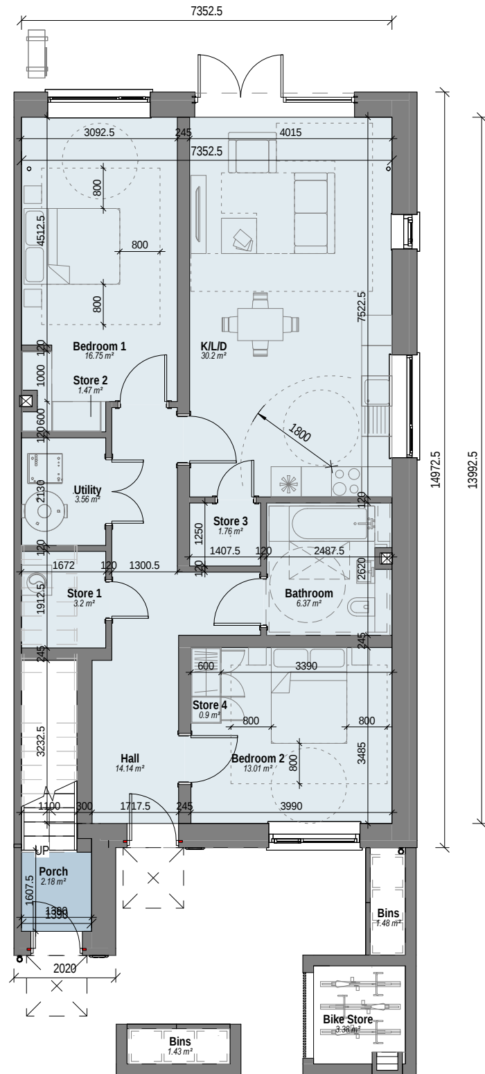
1 DDE - Level 00 Scale: 1 : 100
